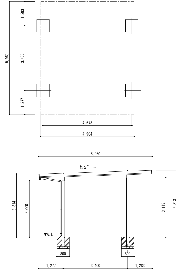
■ 基礎配置図
