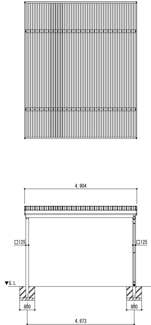
■ 立面図
